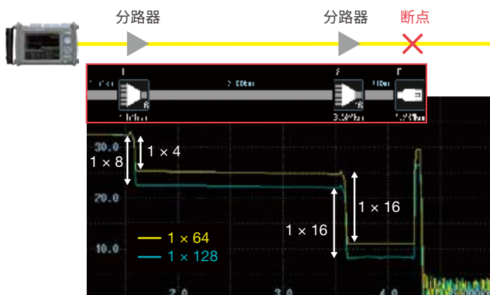
通过128和64端口分路器的测量实例
