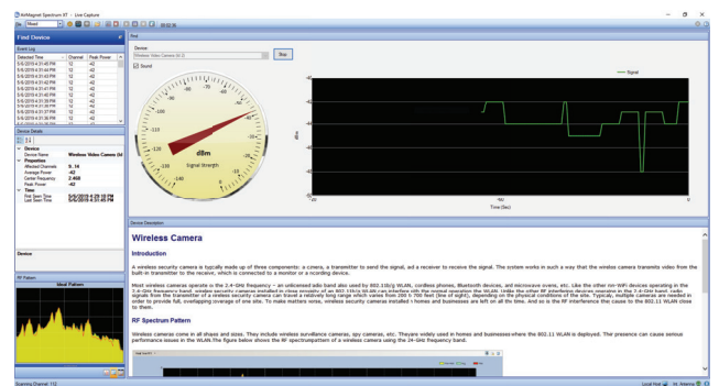
自动检测任何射频干扰源
