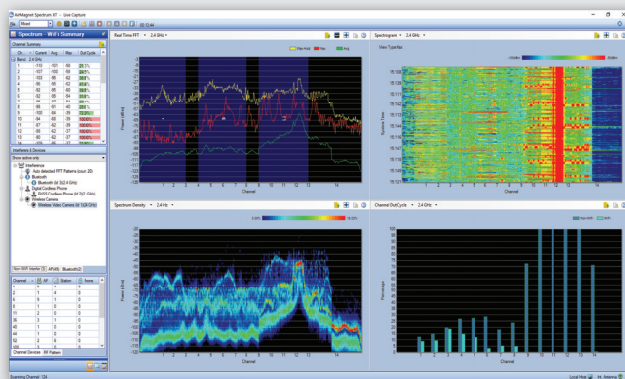
射频频谱诊断视图
