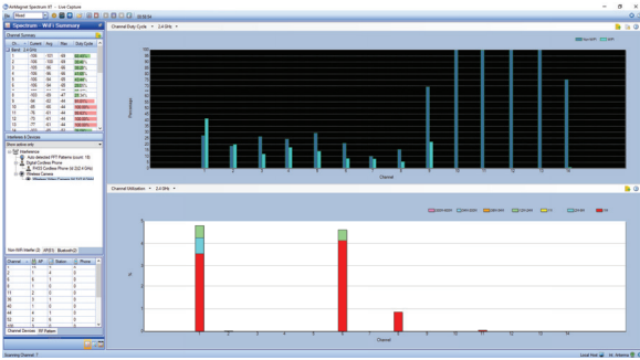
射频干扰和 WiFi 影响分析
